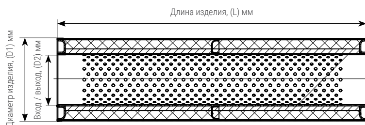
Чертеж пламегасителя универсального двухкамерного с перфорированной трубой
