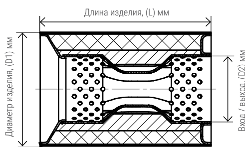
Чертеж пламегасителя коллекторного с формованным диффузором
