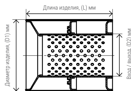
Чертеж пламегасителя коллекторного с перфорированной трубой и диссипативной перегородкой
