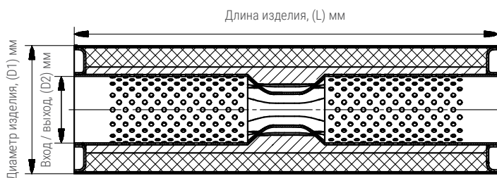
Чертёж пламегасителя универсального однокамерного с формованным диффузором
