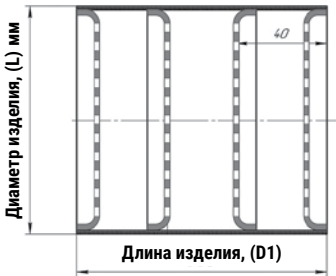
Чертеж пламегасителя коллекторного секционного ZeroNoise
