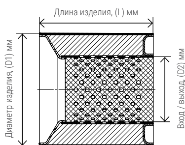
Чертеж пламегасителя коллекторного с перфорированной трубой
